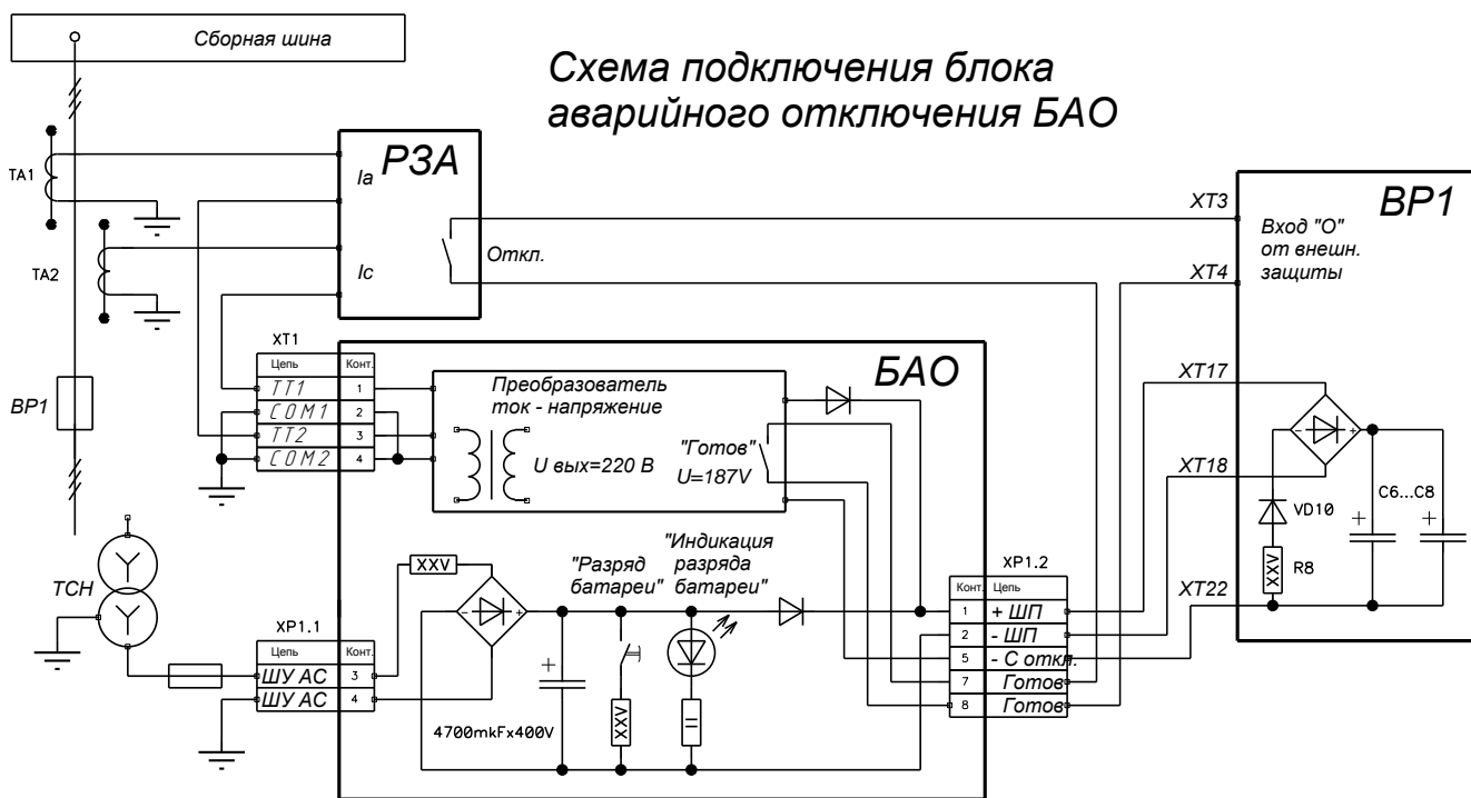
Рис.2. Схема подключения БАО
